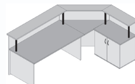
Primjer složenog pulta 247x172x110h
